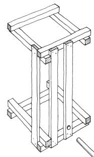
Fig. 53 b Stativet er bygd av høvlede lister: 1,2 m av 15x15 mm 3,6 m av 8x22 mm + en rundstokk: 8 mm i diameter
