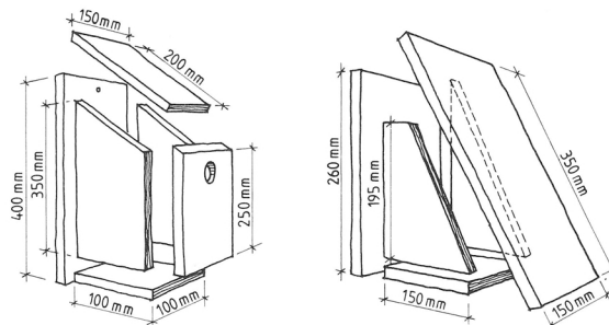
Fig. 31 a Dimensjoner på fuglekasse
