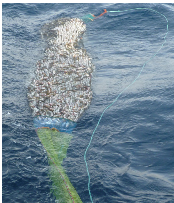
Bilde 2-6; Hiving av not i overflateposisjon. Foto: SINTEF Fiskeri og havbruk AS
