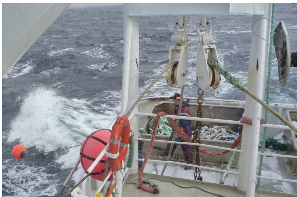
Bilde 2-5; Setting av snurrevad. Foto: SINTEF Fiskeri og havbruk AS
