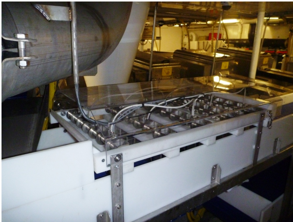
Bilde 2-3; Elektrobedøver integrert i produksjonslinja. Foto: SINTEF Fiskeri og havbruk AS
